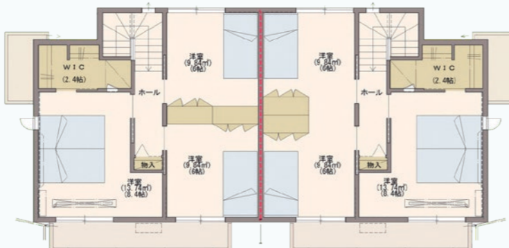
2階間取り図
