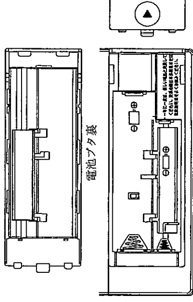
＜本体＞図3-2 単一、単三電池使用の場合
